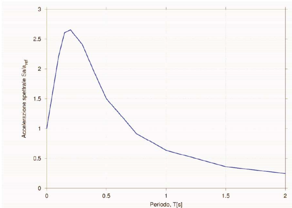
Figura 1: Spettro di risposta normalizzato (Periodo di ritorno: 475 anni, smorzamento: 5%) l'Emilia-Romagna
