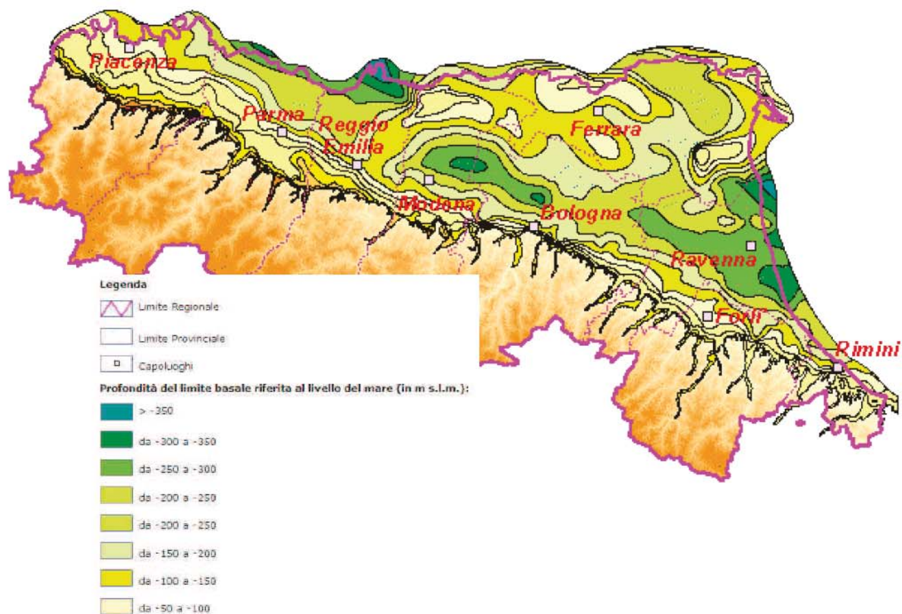
Profondità del limite basale del Gruppo Acquifero "A" (RER)
