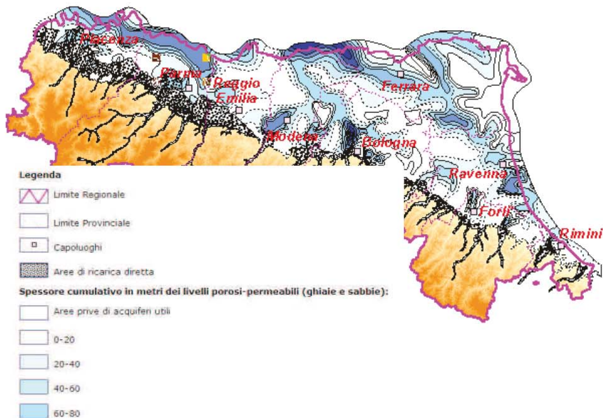
Depositi poroso permeabili del Gruppo acquifero "A" (RER)
