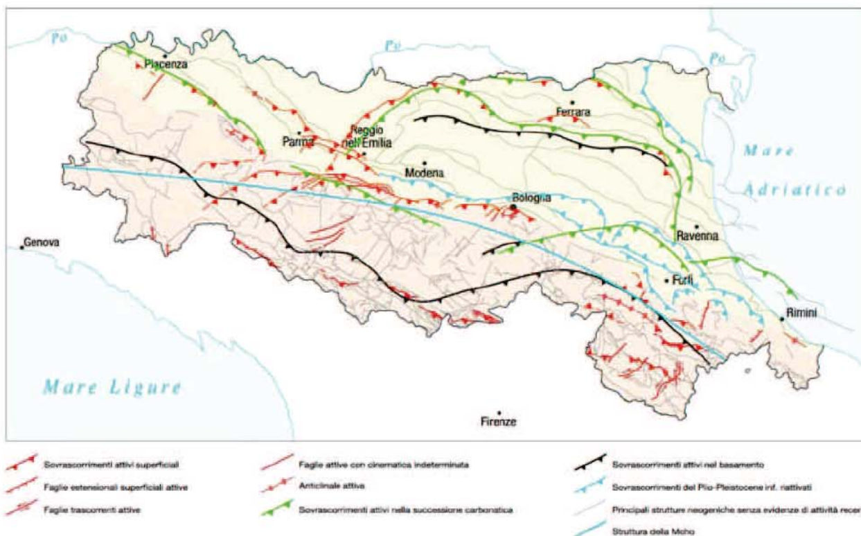
Figura 1 - Attività neotettonica in Emilia-Romagna (da: "Note illustrative - Carta Sismotettonica della Regione Emilia-Romagna" - Servizio Geologico Sismico e dei Suoli - Regione Emilia-Romagna - 2004)
