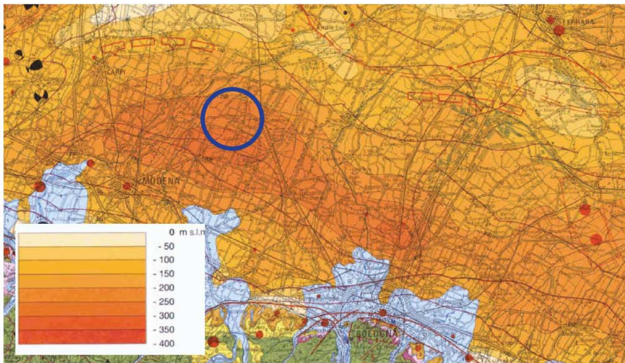
CARTA SISMOTETTONICA DELLA REGIONE EMILIA-ROMAGNA
